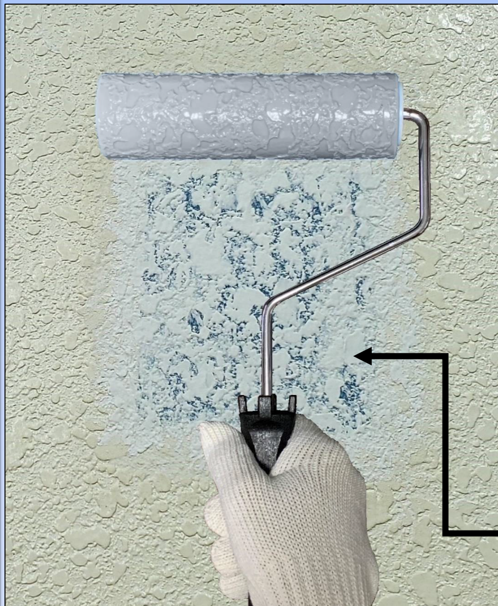
魔法ローラーF(吹放し玉模様)
